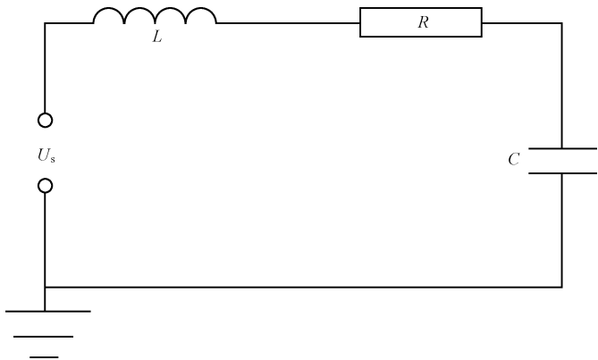
图 B.1 调感式串联谐振试验回路
